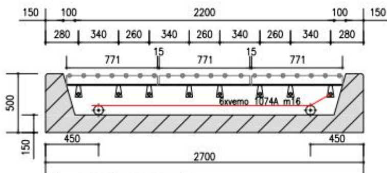
Dwarsdoorsnede
