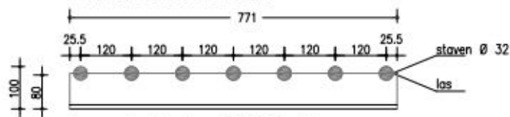
Aanzicht L 80.80.10
