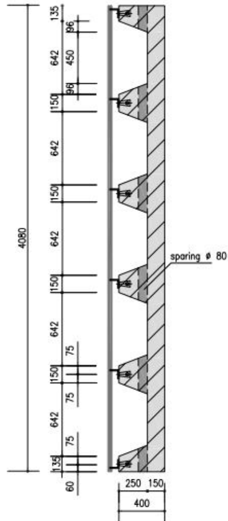
Langsdoorsnede
