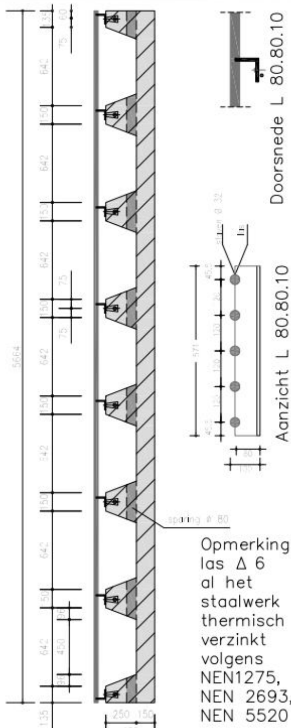
Langsdoorsnede
