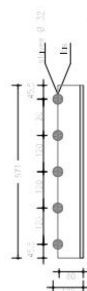
Aanzicht L 80.80.10
